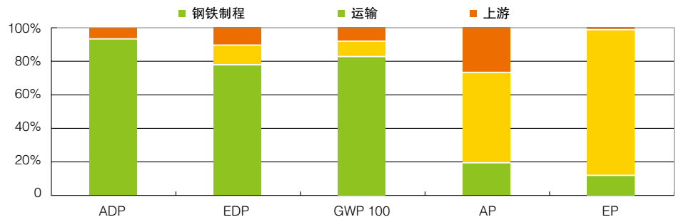
图 1 1kg 电镀锌产品生命周期各阶段对环境影响的相应贡献
